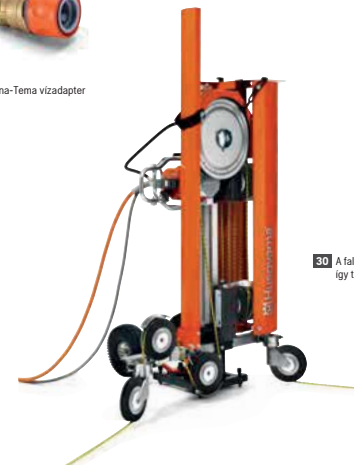
29 Szállítókosci WS 220-hoz
