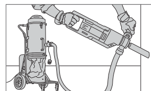
Száraz kézi fúrás.
