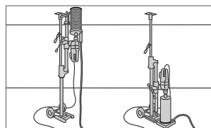
Függőleges fúrás, felfelé és lefelé.
