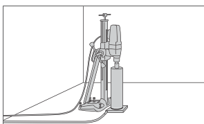
Függőleges fúrás.
