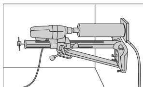
Fúrás csatornák, csövek és kábelek részére.
