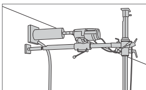
Vízszintes fúrás.
