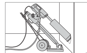
Ferde fúrás.
