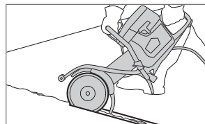
Dilatációs hézagok és repedések homnyainak vágása.
